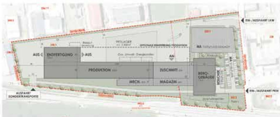
Lageplan der neuen Firmenzentrale
